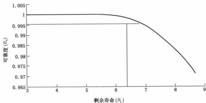
图 F.1 可靠度 R_s 与剩余寿命 R_L 的关系曲线
