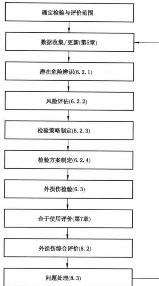
图 1 基于风险的外损伤检验评价流程图
