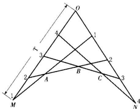
图 A.2.1 “工兵法”放样
