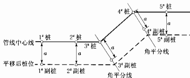
图 5.2.2 平原地区移桩方法
