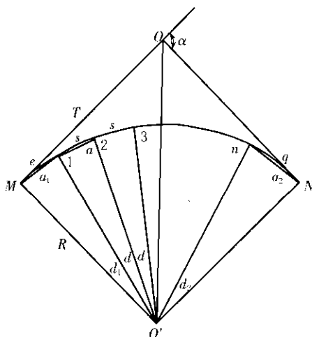
图 A.2.3 “总偏角法”放样
